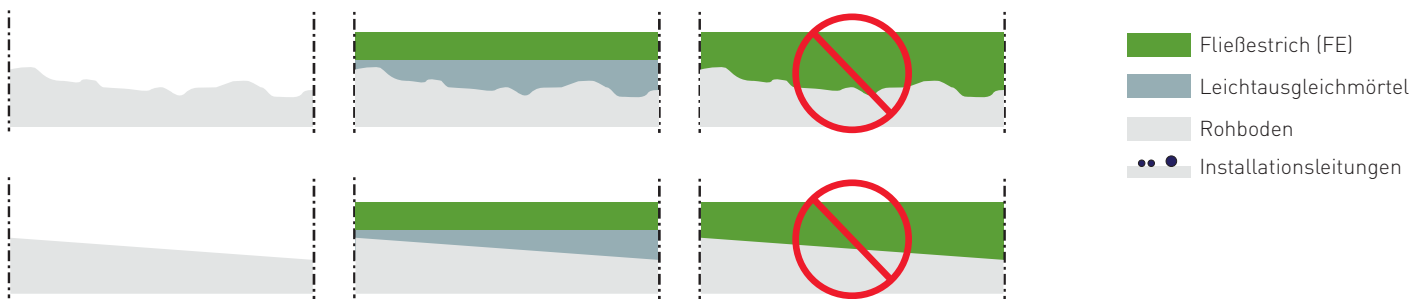
Abb. 2: Beispiel Ausführungsskizzen „Unebene und schiefe Oberflächen der Rohdecken bzw. -böden“
